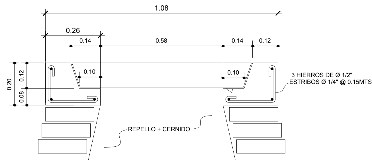
DETALLE DE TAPADERA Y BROCAL ESC. 1/10
