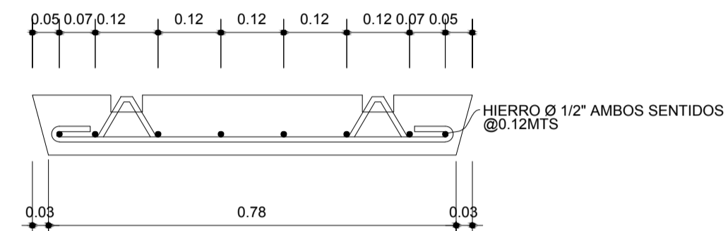
SENCIÓN C-C' ESC. 1/10
