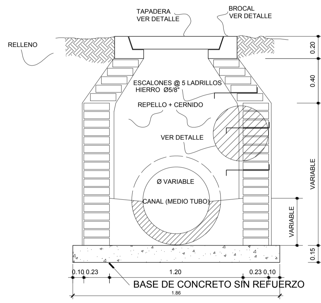
SECCION A ESC. 1/20
