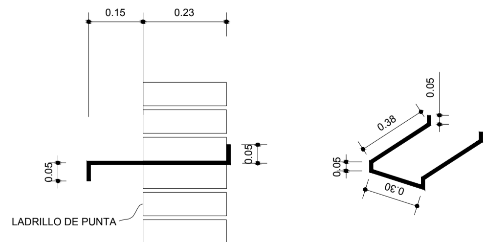
DETALLE DE ESCALÓN ESC. 1/10
