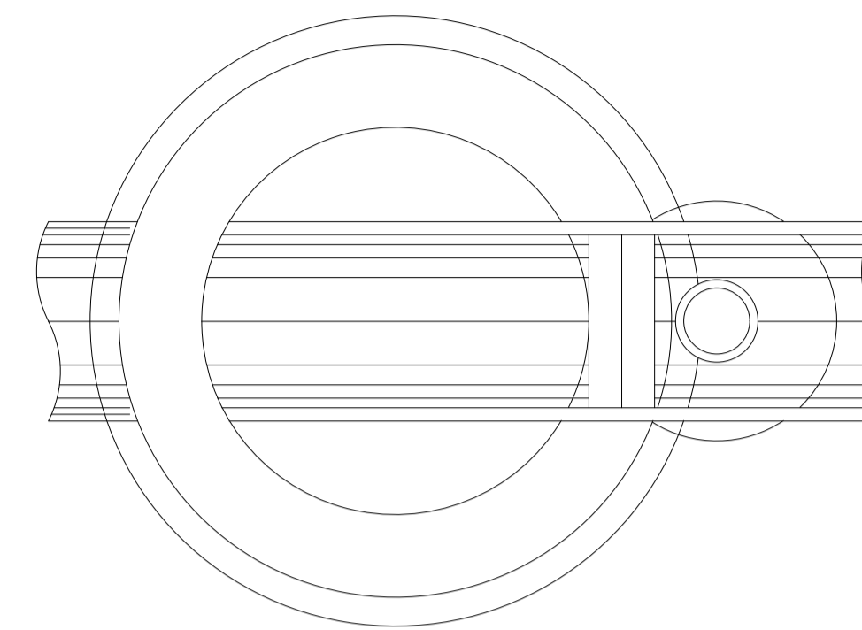
PLANTA G-G' ESC. 1/20
