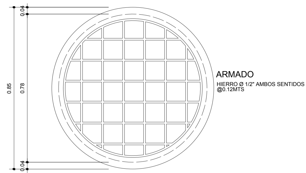
PLANTA TAPADERA ESC. 1/10
