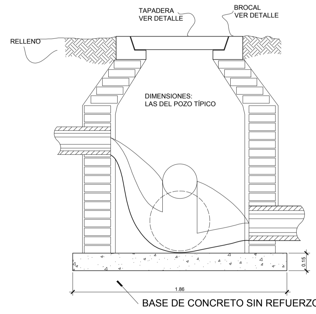
SECCION A ESC. 1/20
