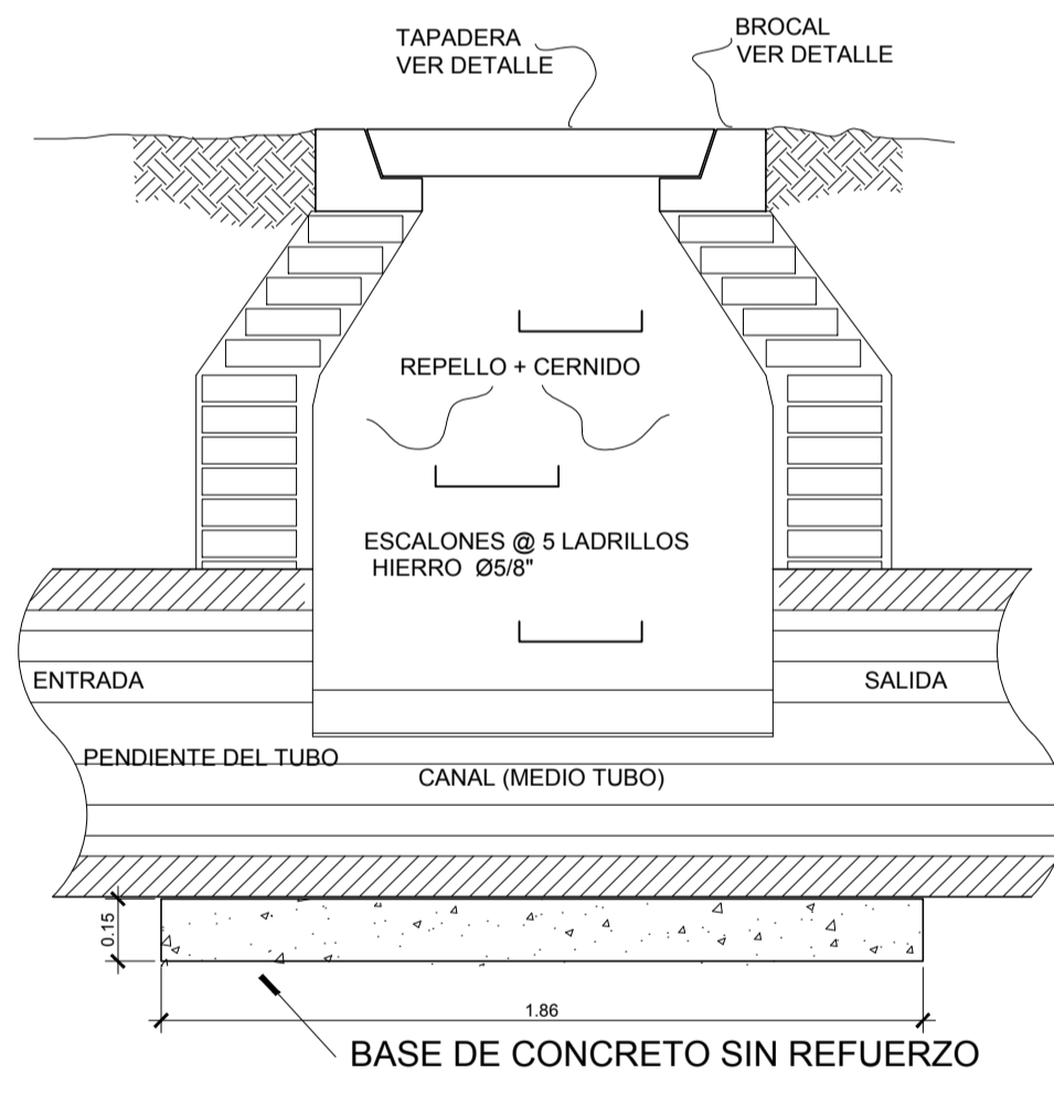
SECCION A ESC. 1/20
