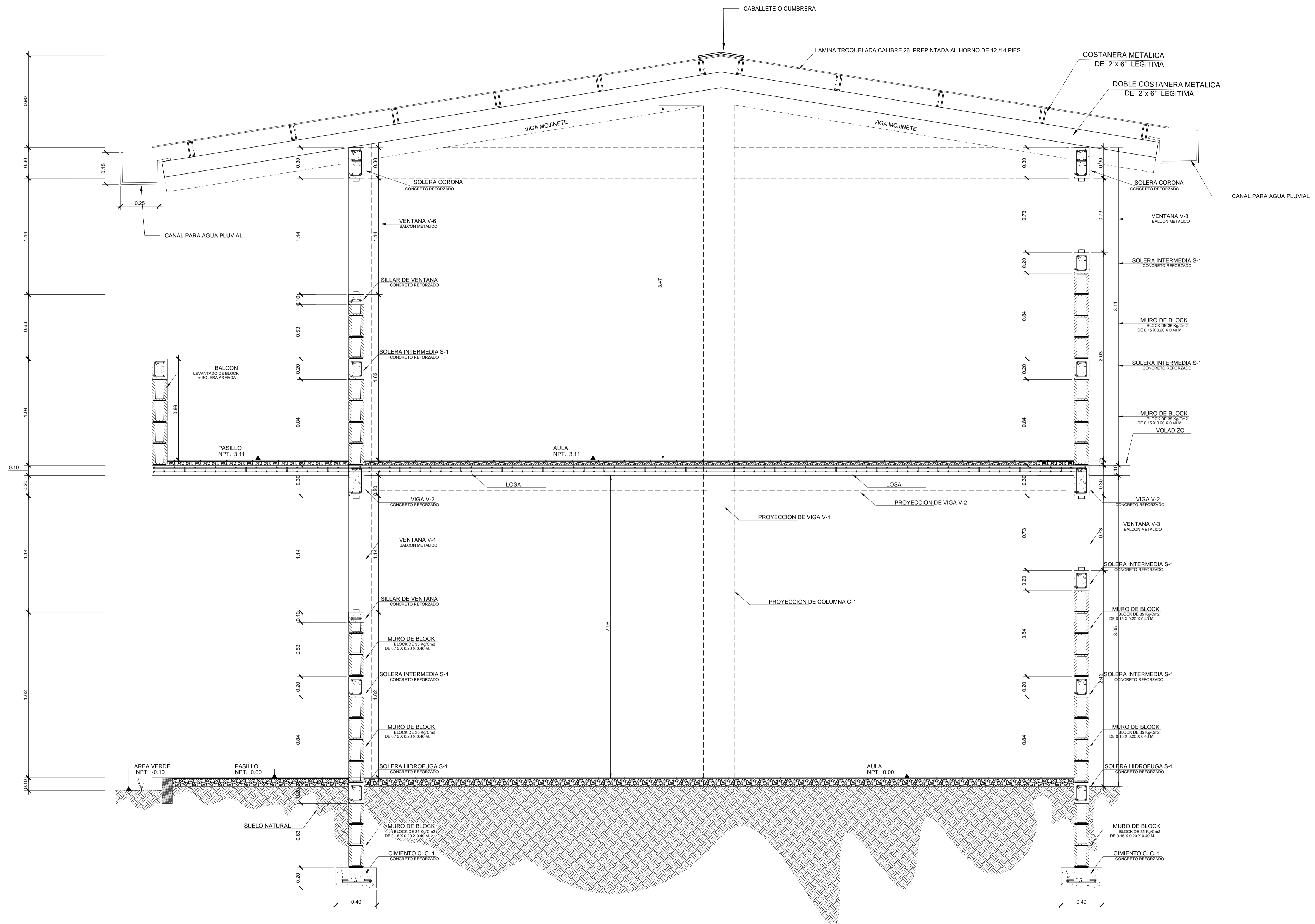
DETALLE DE CORTE B - B' ESCALA 1 : 20
